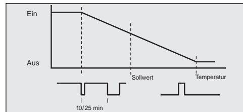
Bild 1: Verlauf der relativen Einschaltdauer (Tastverhältnis) in Abhängigkeit von der Temperatur
